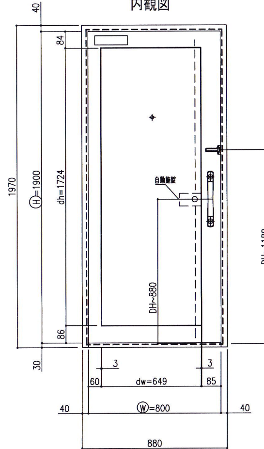
内観図
