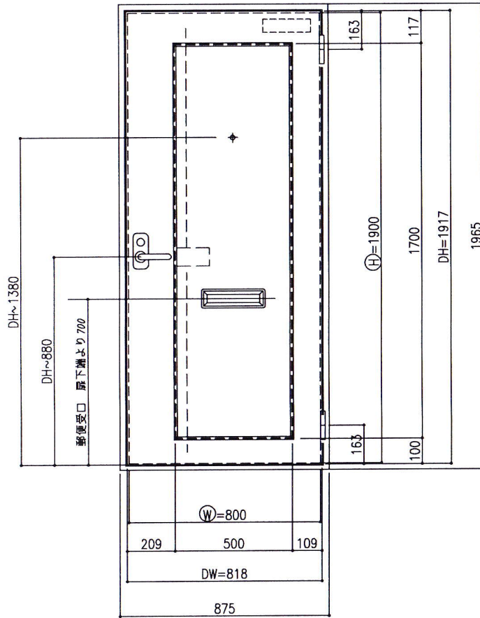
外観図
